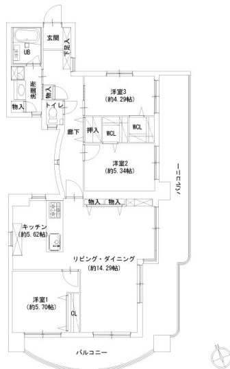
間取図
