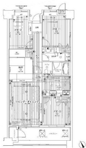
間取図
