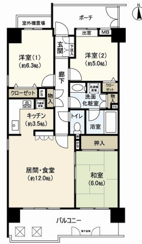
間取図
